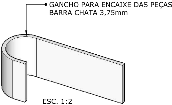
ESC. 1:2
