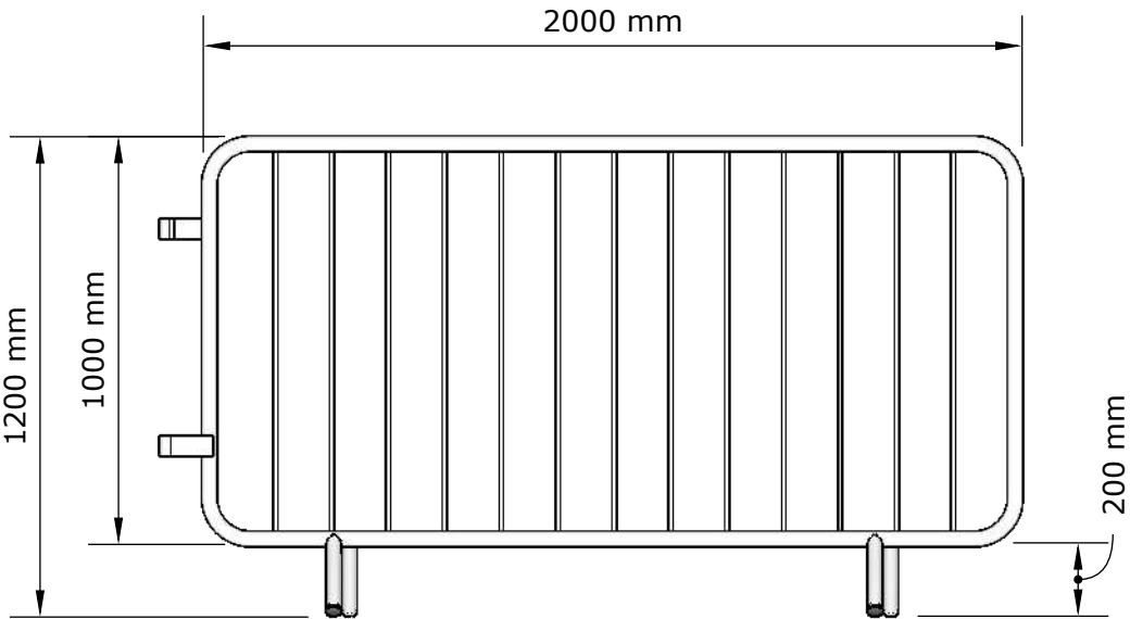
ESC. 1:20
